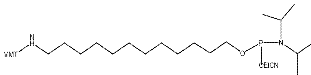
MMT: 4-Monomethoxytrityl
