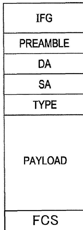
FIG. 2A
