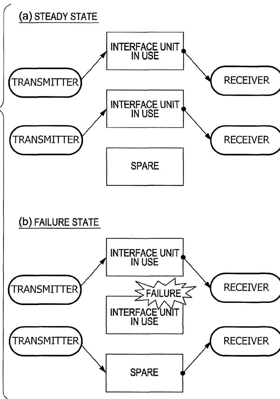
FIG. 13C
