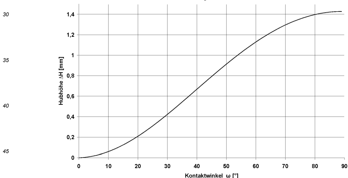
Hubhöhe \Delta H des Aufbauteils mit einem elliptischen angeformten Kontaktstift in einer elliptisch angepassten Formausnehmung im Pfostenteil bei einem rotatorischen Kontaktwinkelsatz \omega um die Achse des angeformten Kontaktstifts
