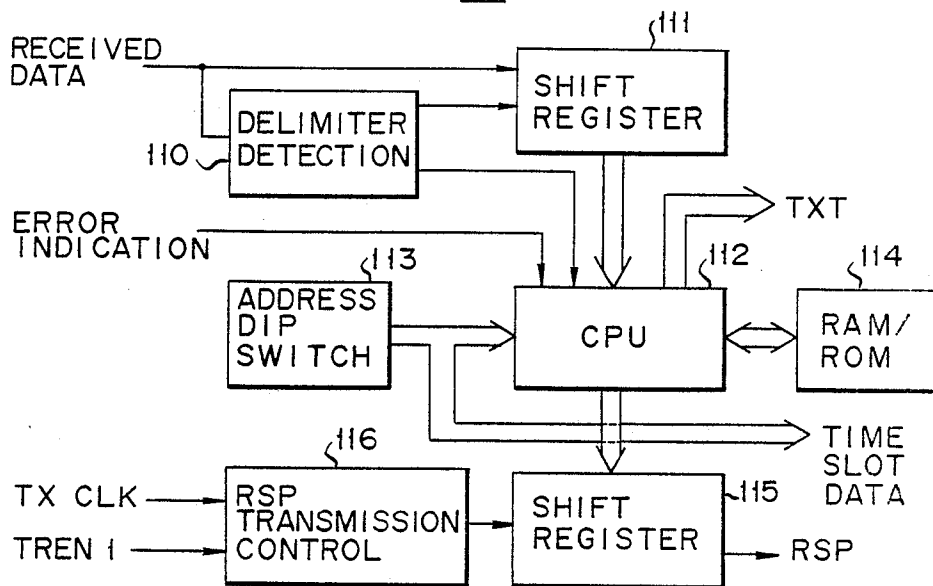
ASG/RSP PROCESSING MODULE 94
