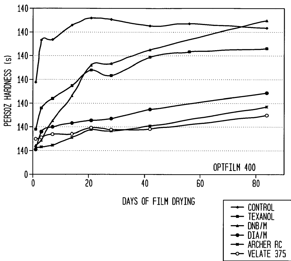
FIG. 12 PERSOZ HARDNESS
