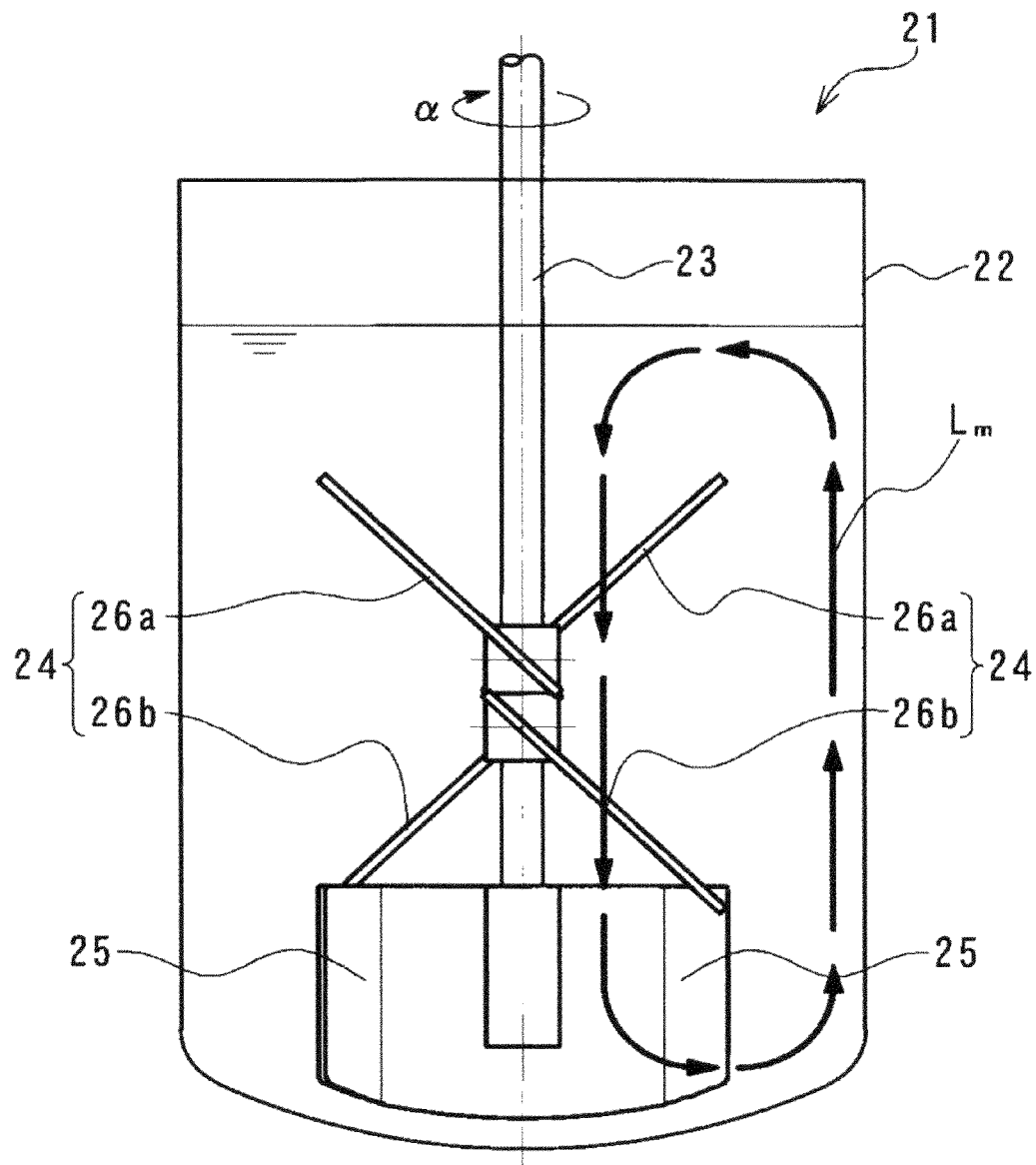
Fig.29(Prior Art)
