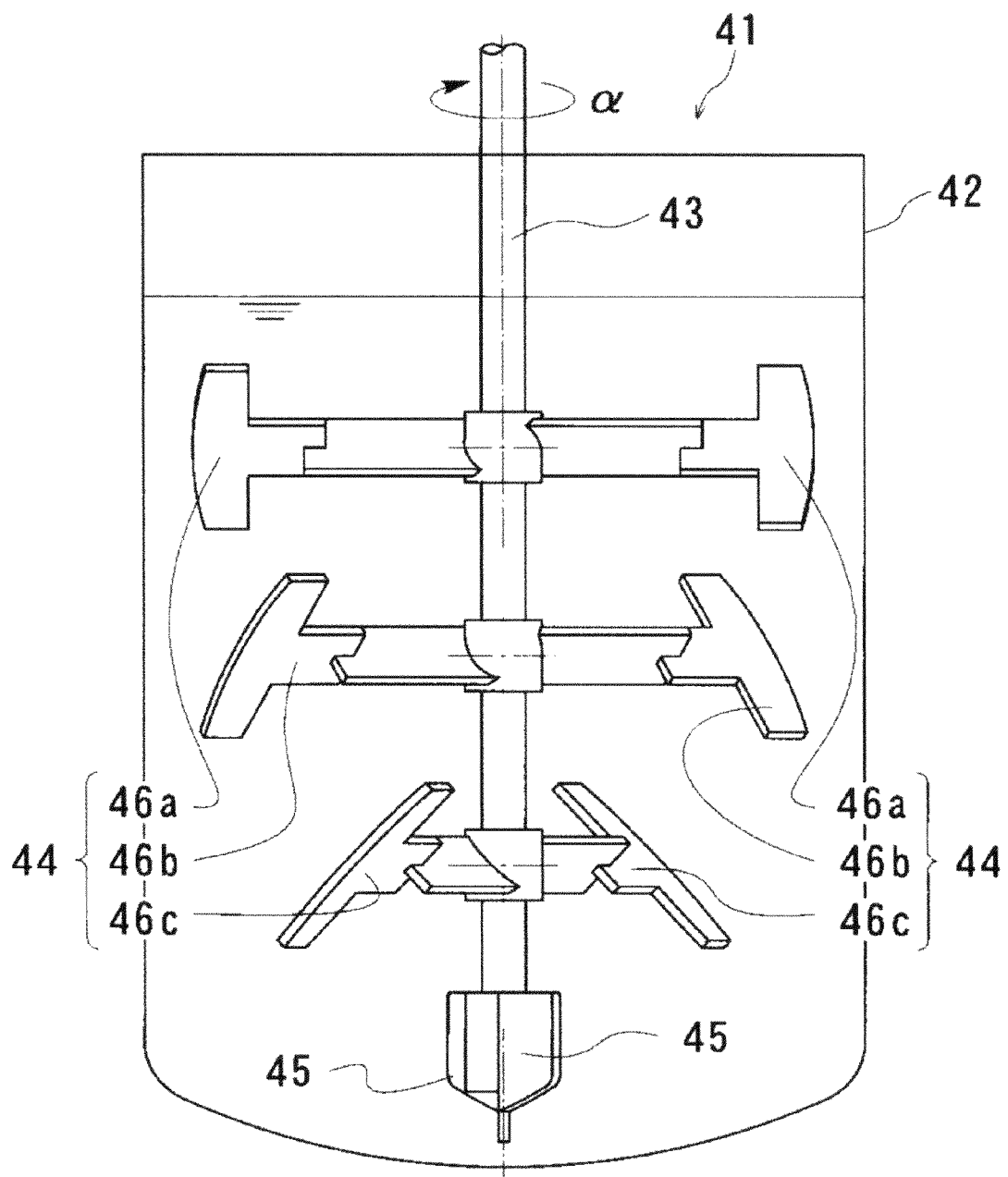
Fig.36(Prior Art)
