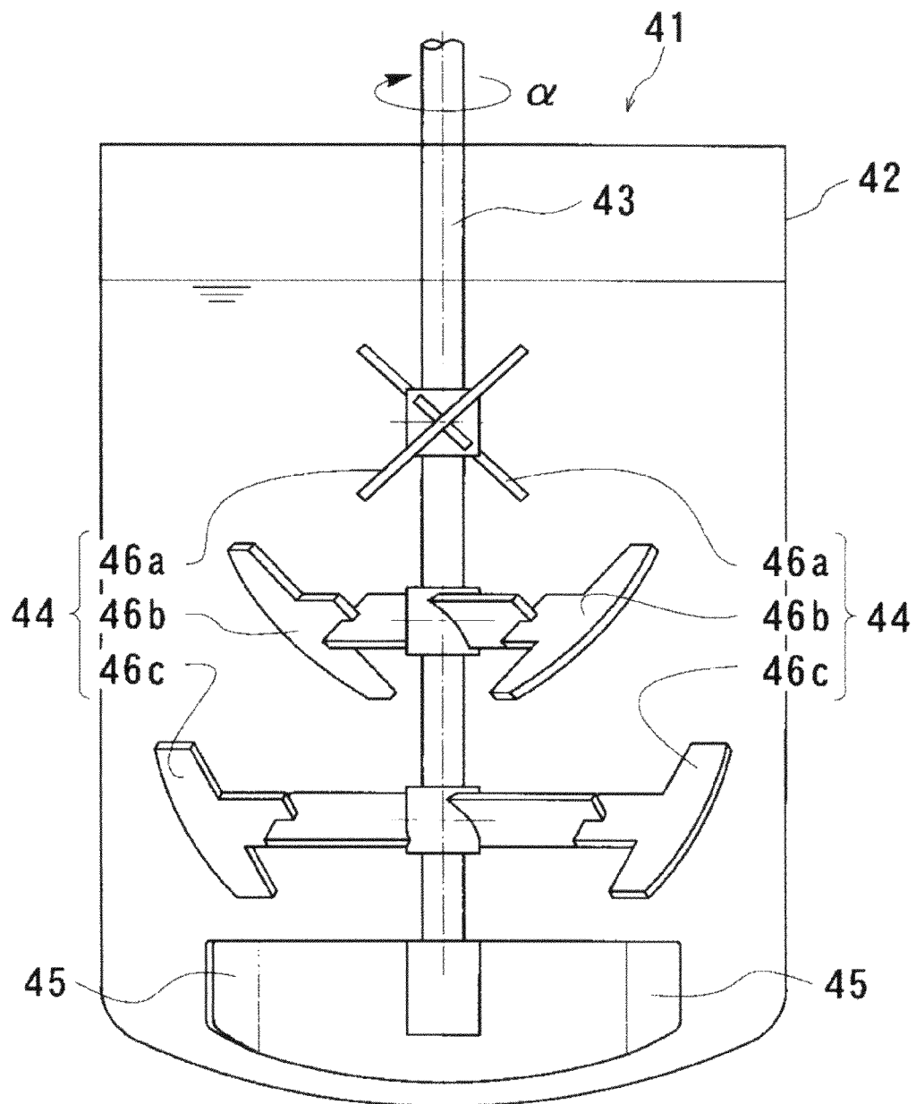
Fig.35(Prior Art)
