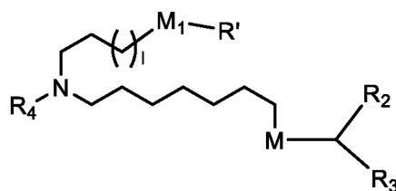
(XI)
