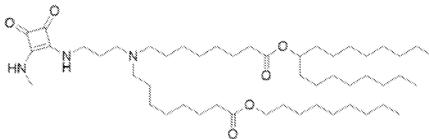
(A4),
