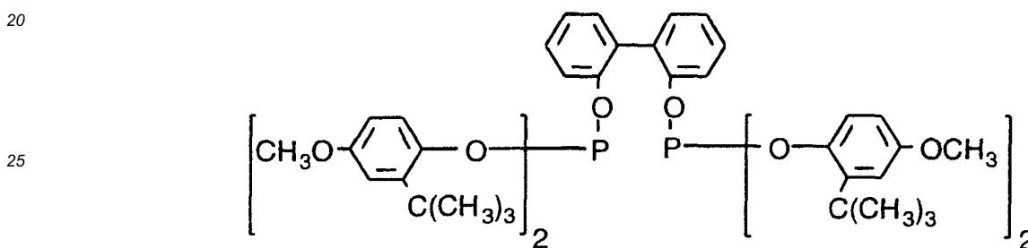
Ligand V
