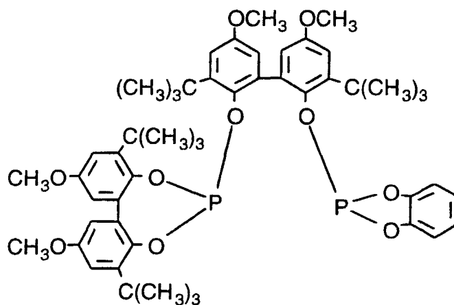
Ligand O
