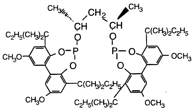
Ligand I
