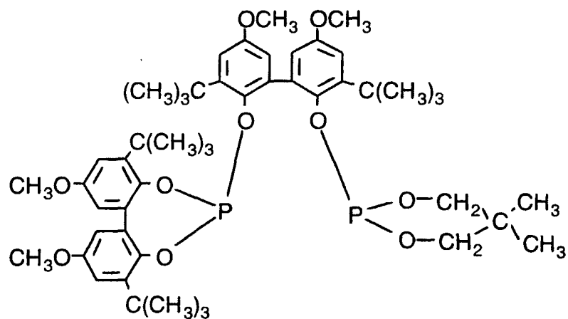
Ligand P
