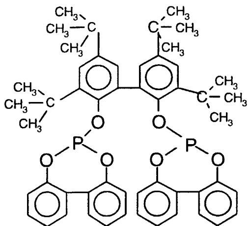
Ligand F
