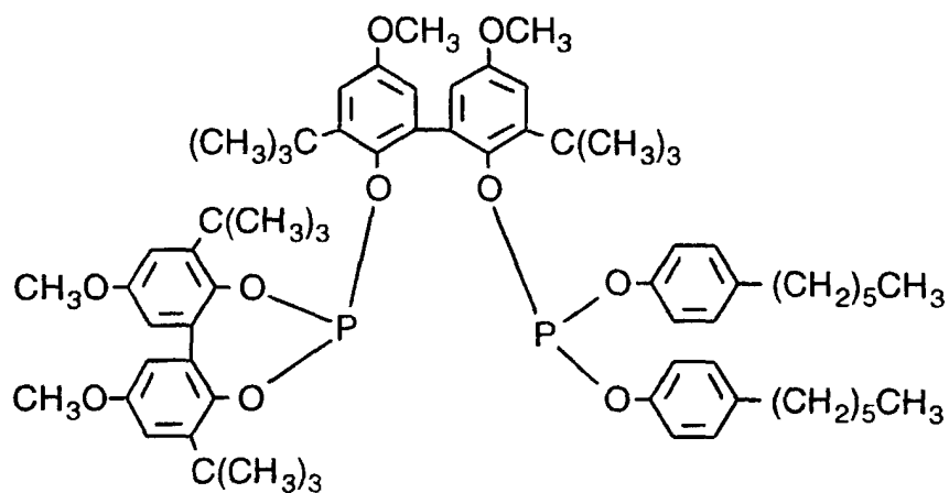
Ligand Q
