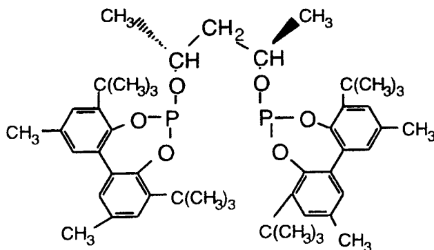
Ligand J
