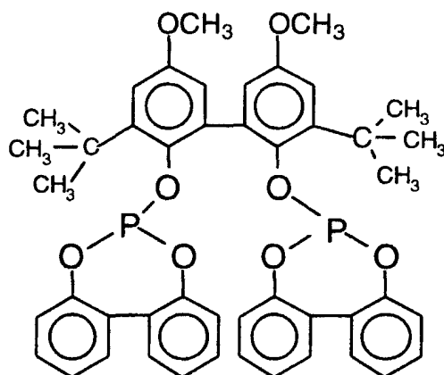
Ligand D
