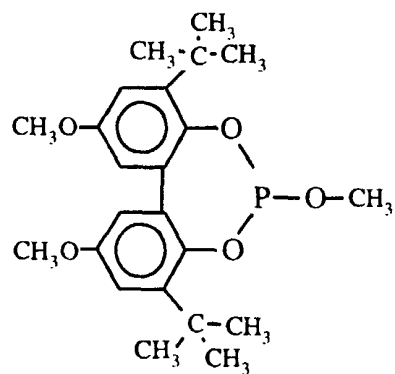
Ligand B
