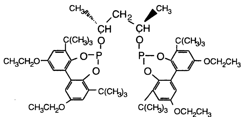
Ligand K
