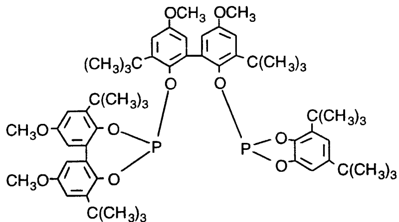
Ligand N
