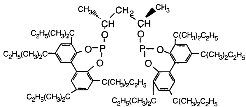
Ligand G
