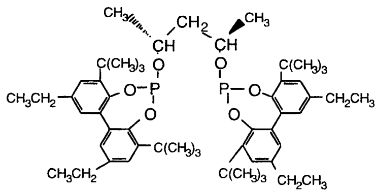
Ligand L
