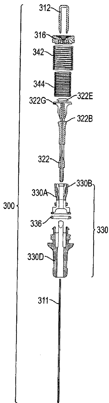
FIG. 9C
