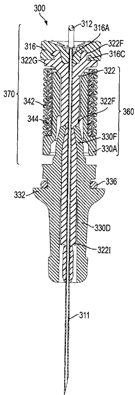
FIG. 9D
