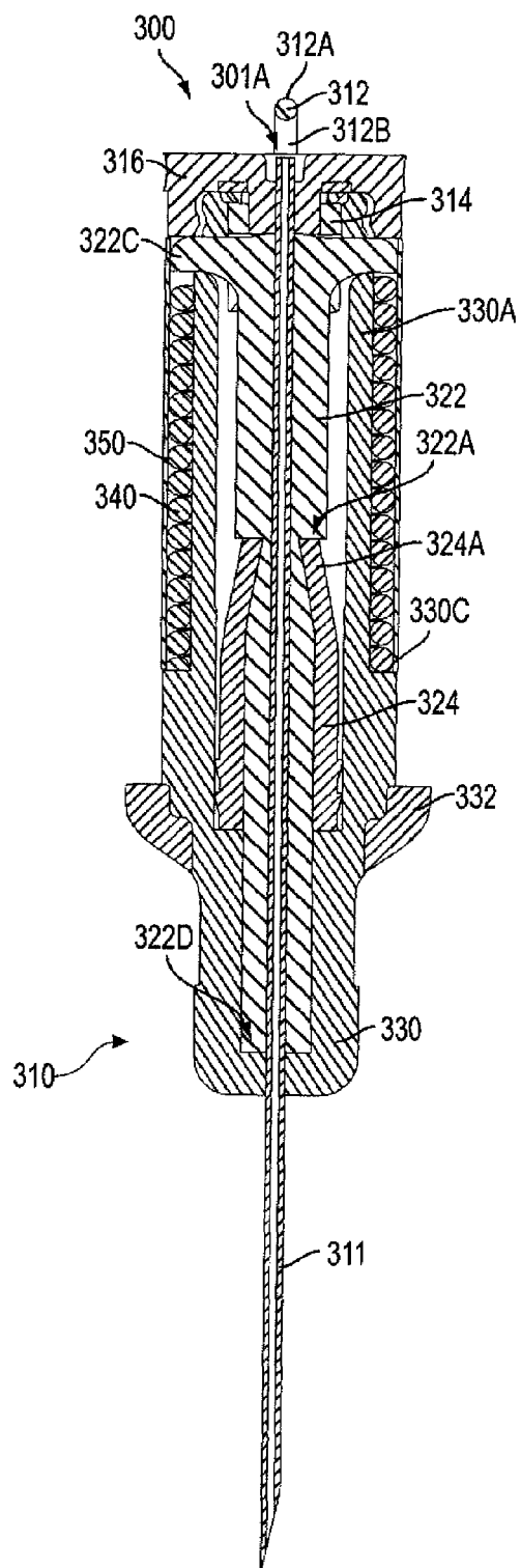
FIG. 9B
