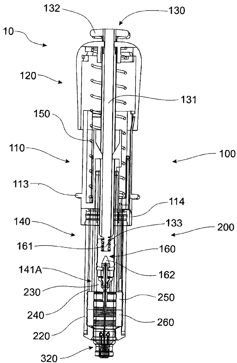
FIG. 10B
