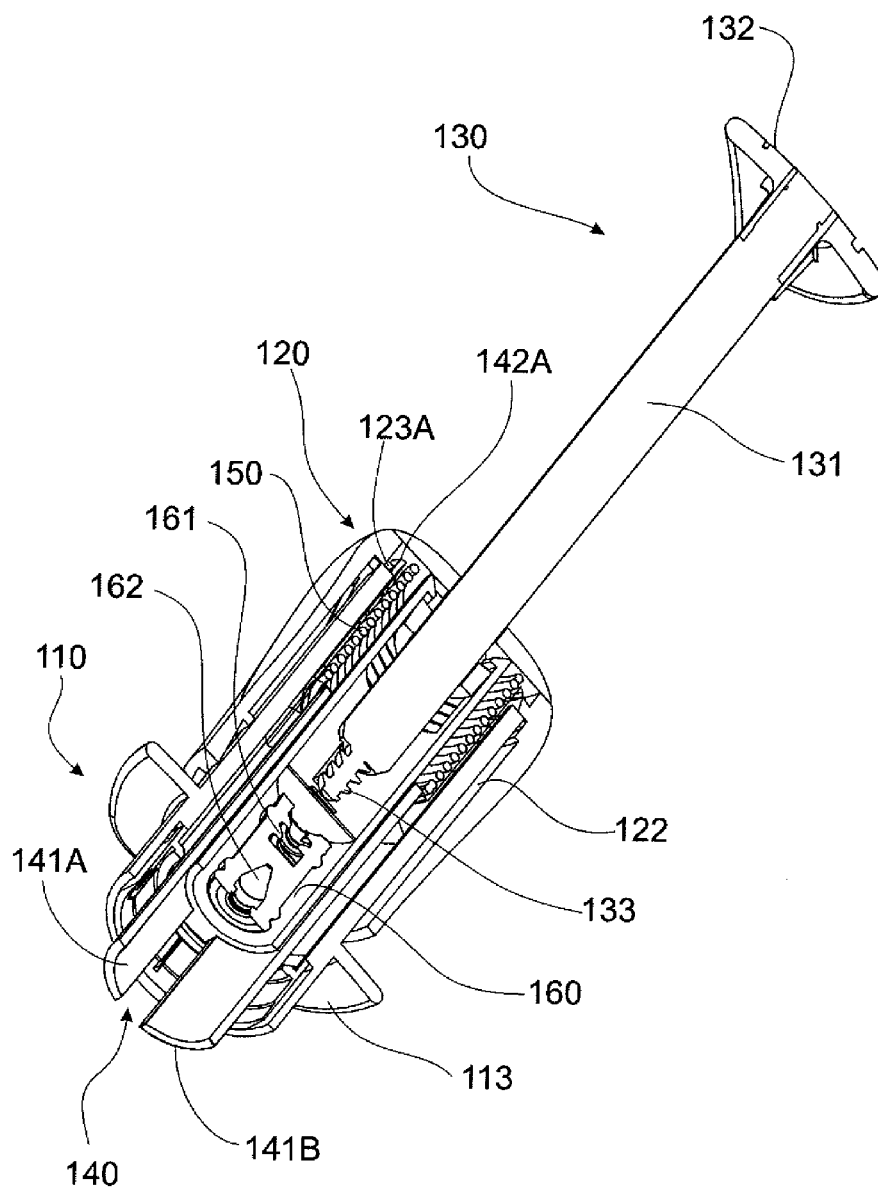
FIG. 3C
