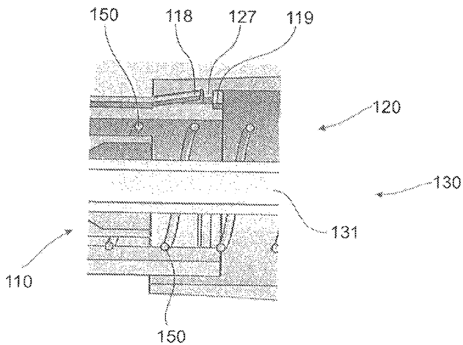
FIG. 10D
