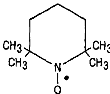
TEMPO
