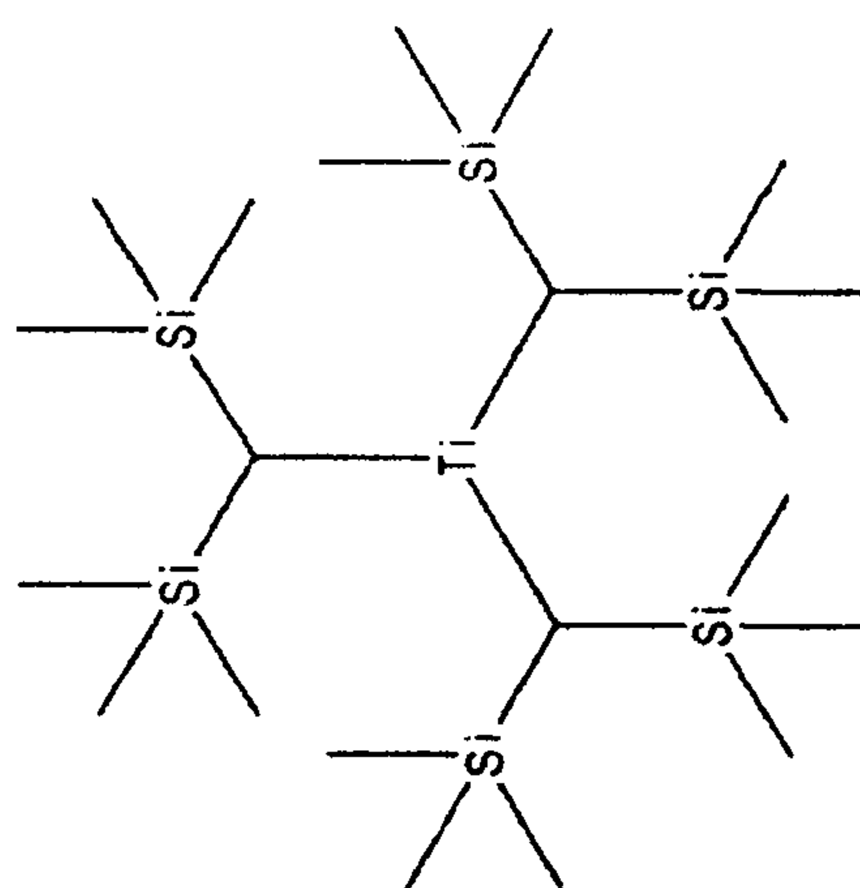
tris [bis(trimethylsilyl)methyl]Titanium
