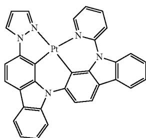
PtN1N
