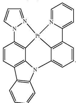
PtN1ppy
