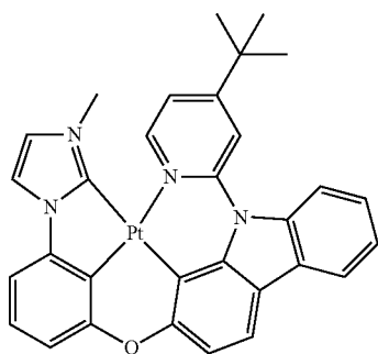
PtON7-t-Bu
