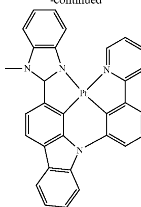
PtN8ppy
