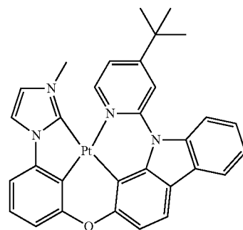
PtON7-t-Bu
