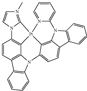
PtN7N
