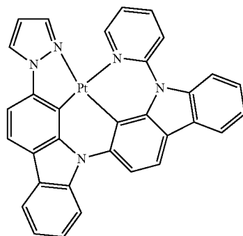
PtN1N
