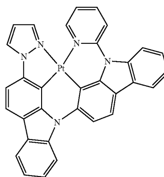
PtN1N
