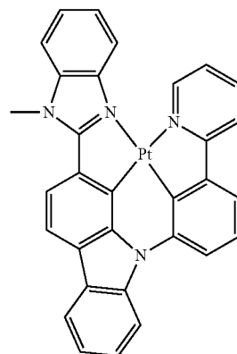
PtN8ppy
