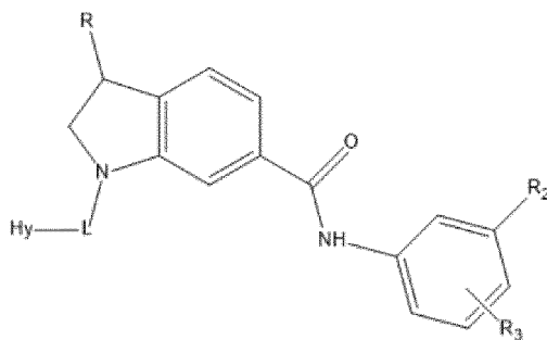
(IAa)
