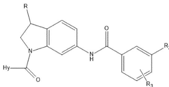
(IBa')
