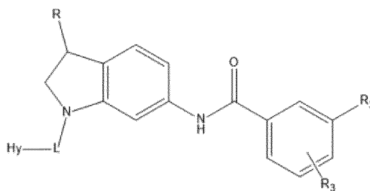
(IBa)
