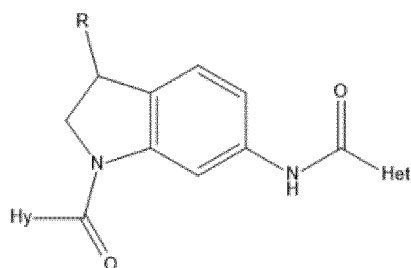
(IBb')
