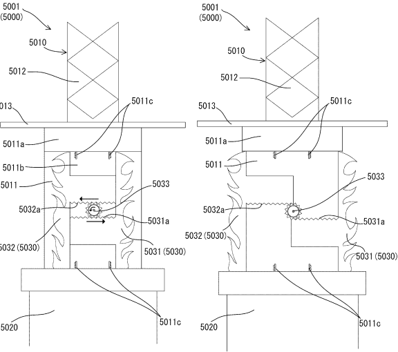
(A) オーラ部材 5030 の閉状態 (B) オーラ部材 5030 の開状態
