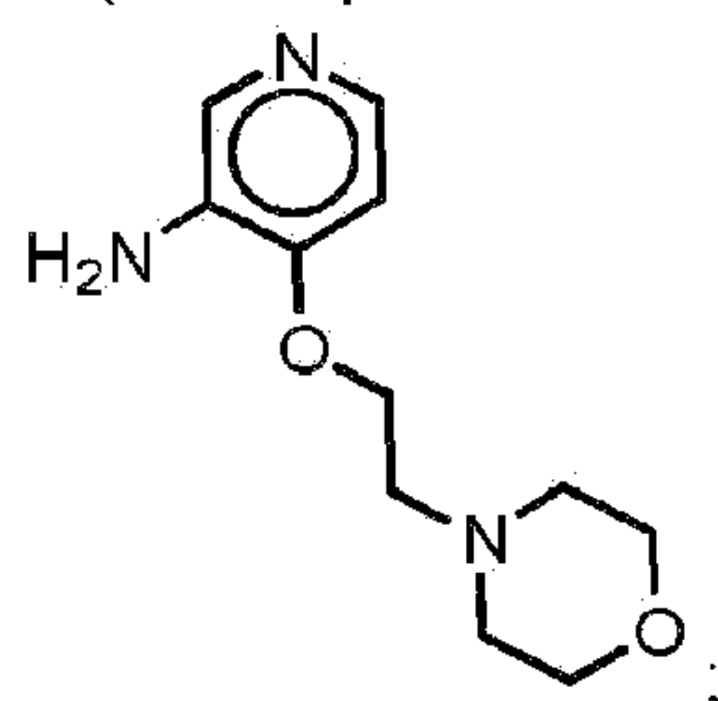
4-(2-morpholinoethoxy)pyridin-3 -amine:
