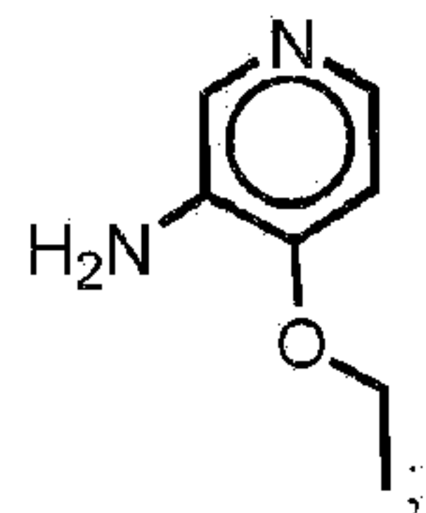
4-ethoxypyridin-3-amine:
