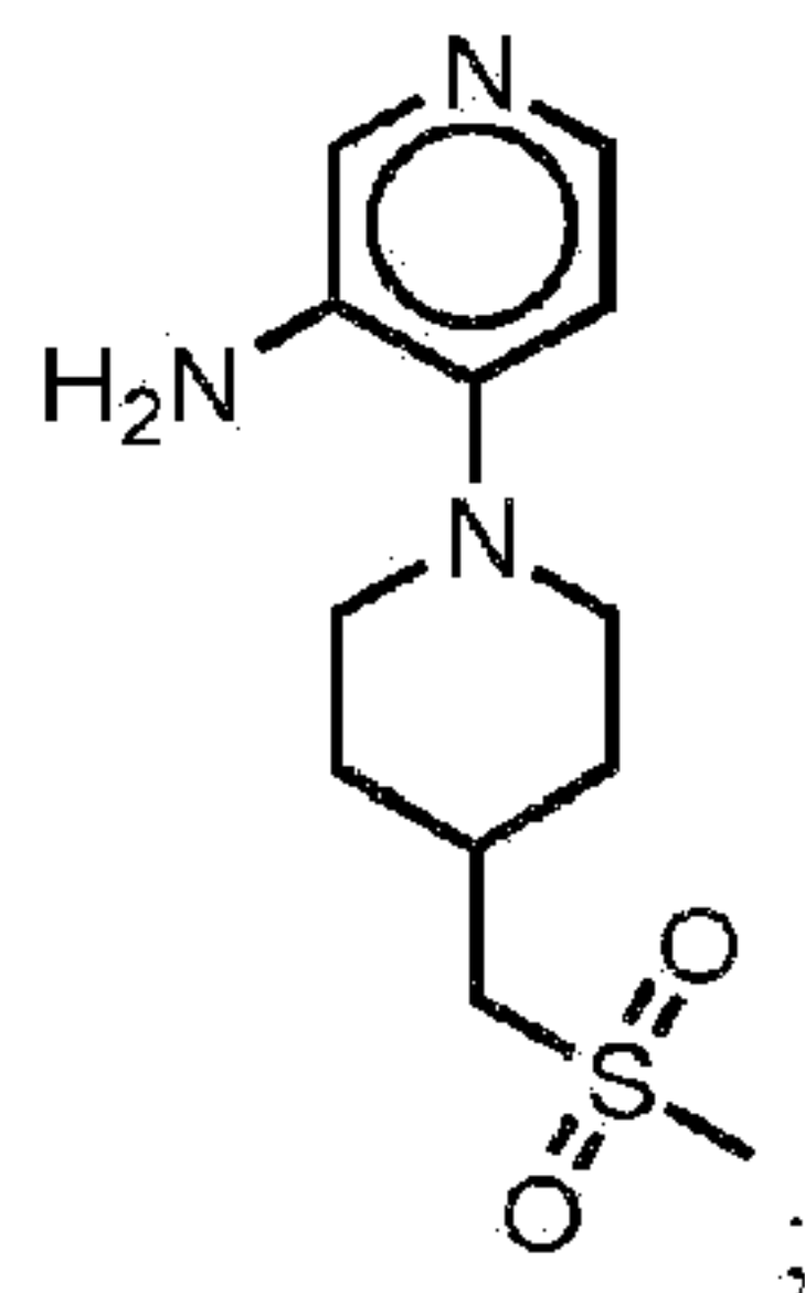
4-(4-((methylsulfonyl)methyl)piperidin-1-yl)pyridin-3-amine:
