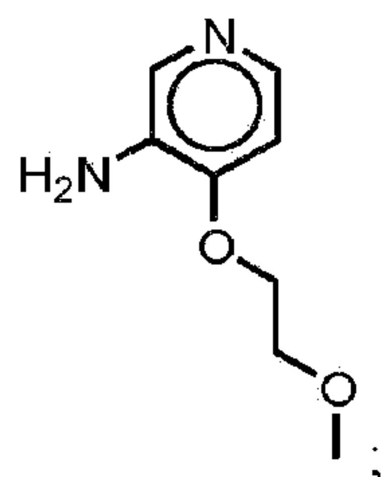
4-(2-methoxyethoxy)pyridin-3 -amine:
