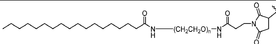
(MAL)-PEG5K+C18
