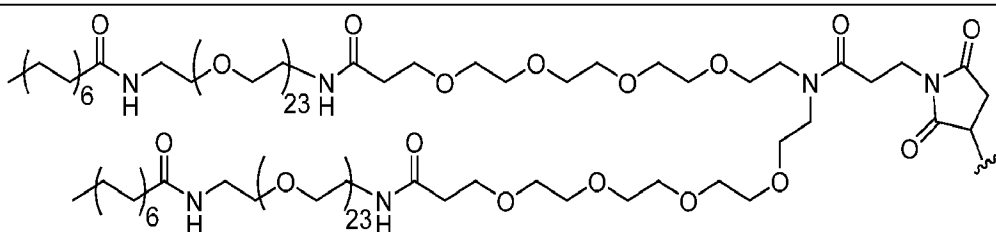
Bis(PEG23+C14)
