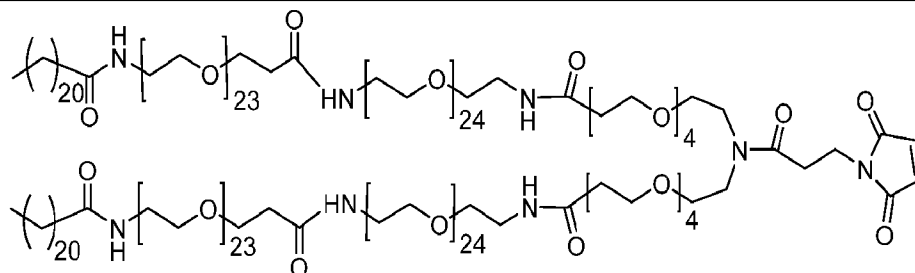
Bis(PEG47+C22)
