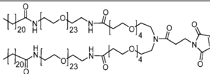
Bis(PEG23+C22)
