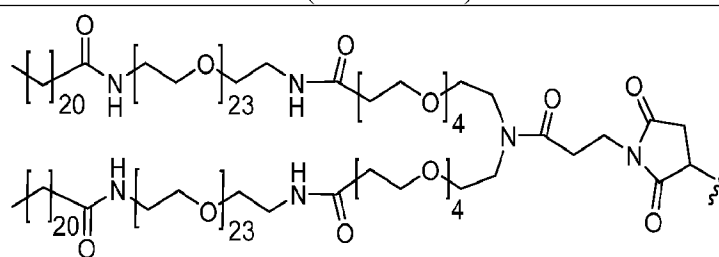
Bis(PEG23+C22)
