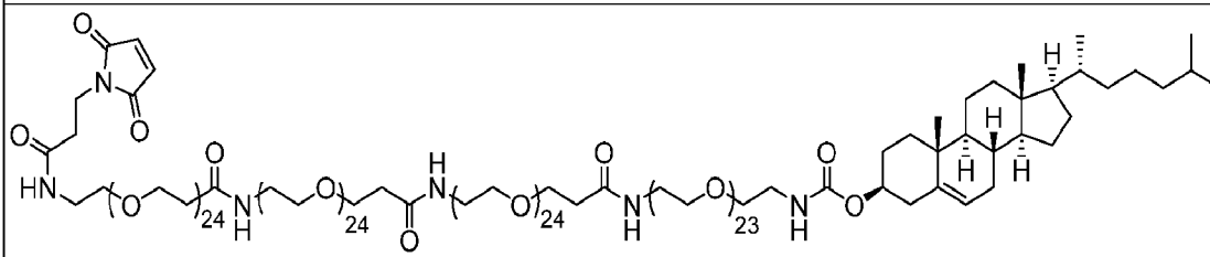
PEG95+CLS
