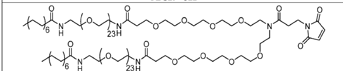
Bis(PEG23+C14)
