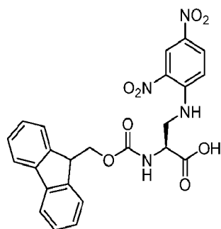
Fmoc-Dap(DNP)-OH
