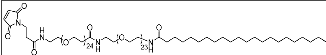
PEG47+C22
