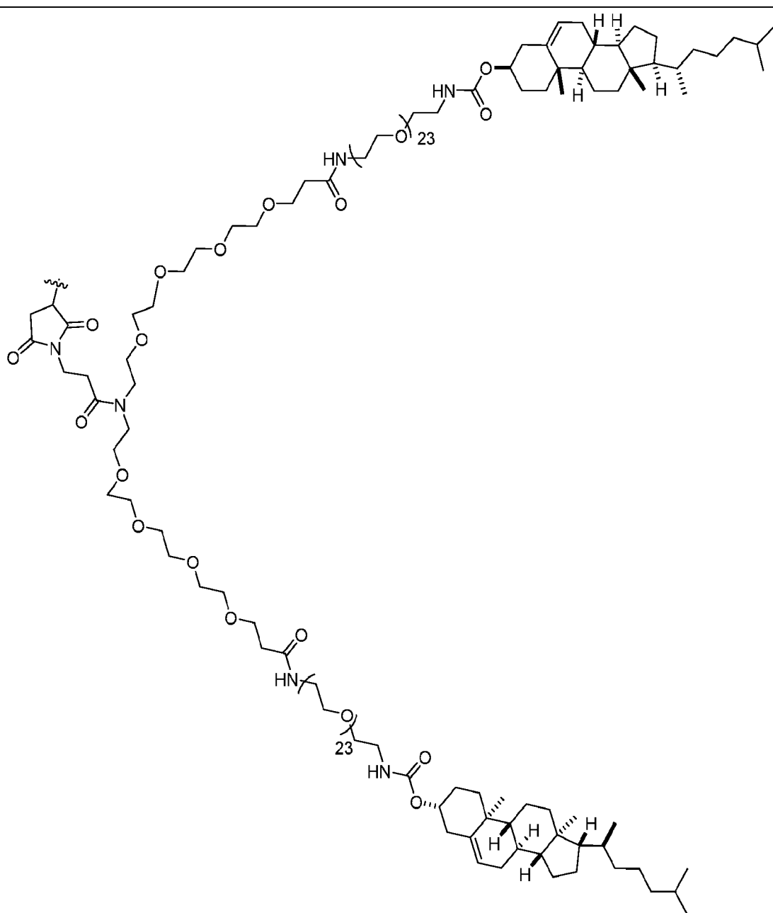
Bis(PEG23+CLS)
