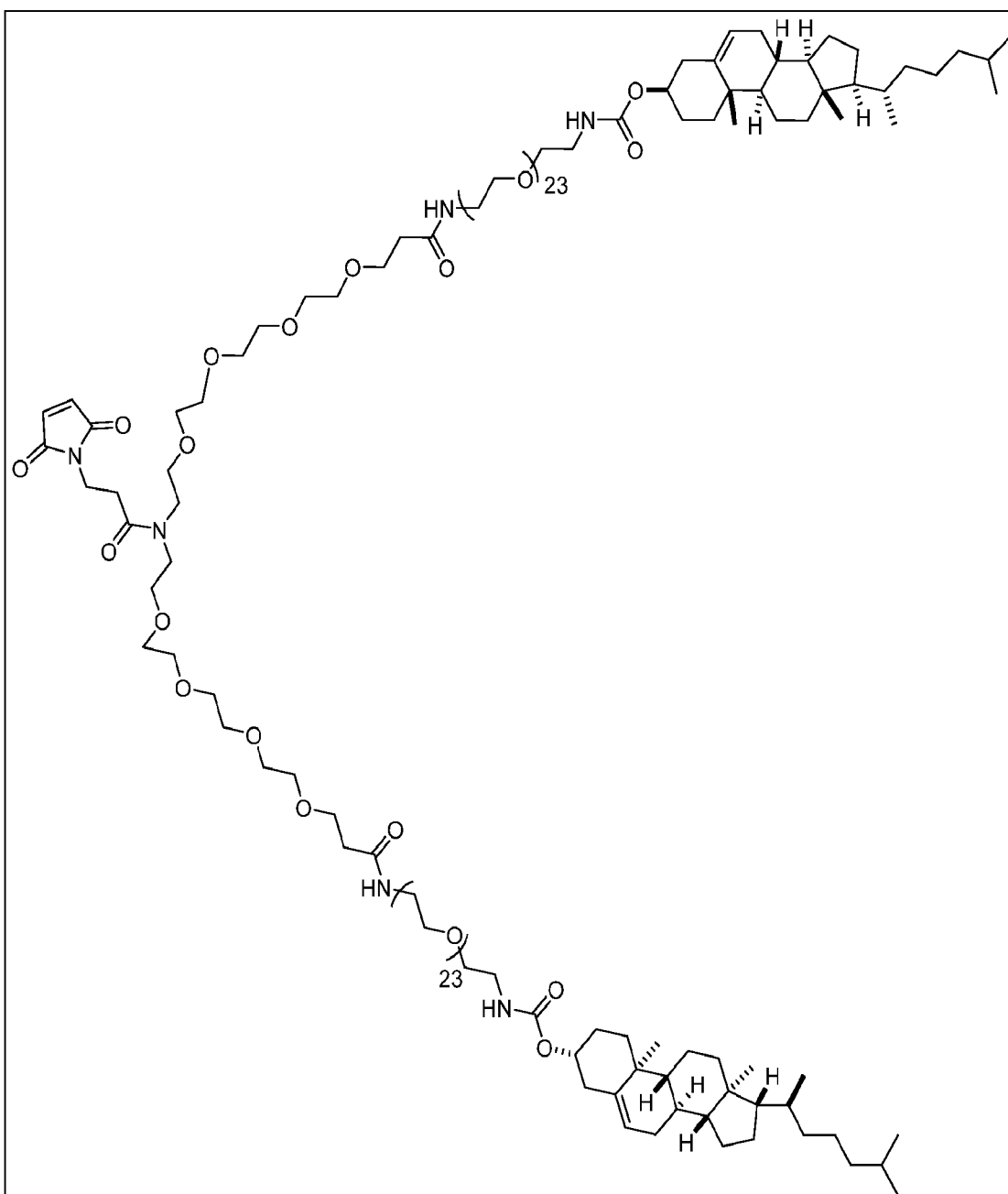
Bis(PEG23+CLS)
