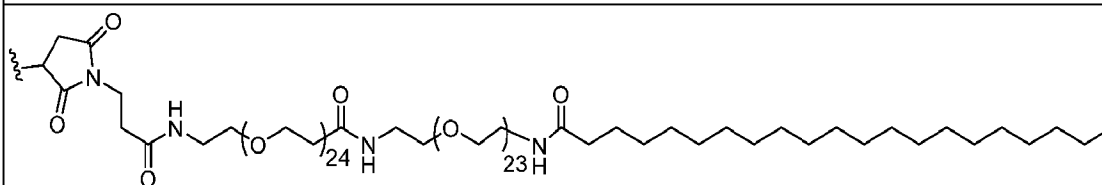
PEG47+C22
