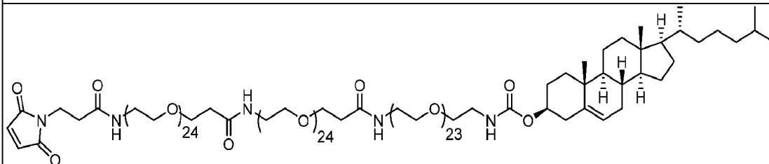
PEG71+CLS
