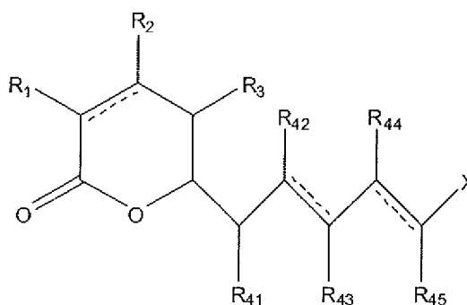
Fragment A:
