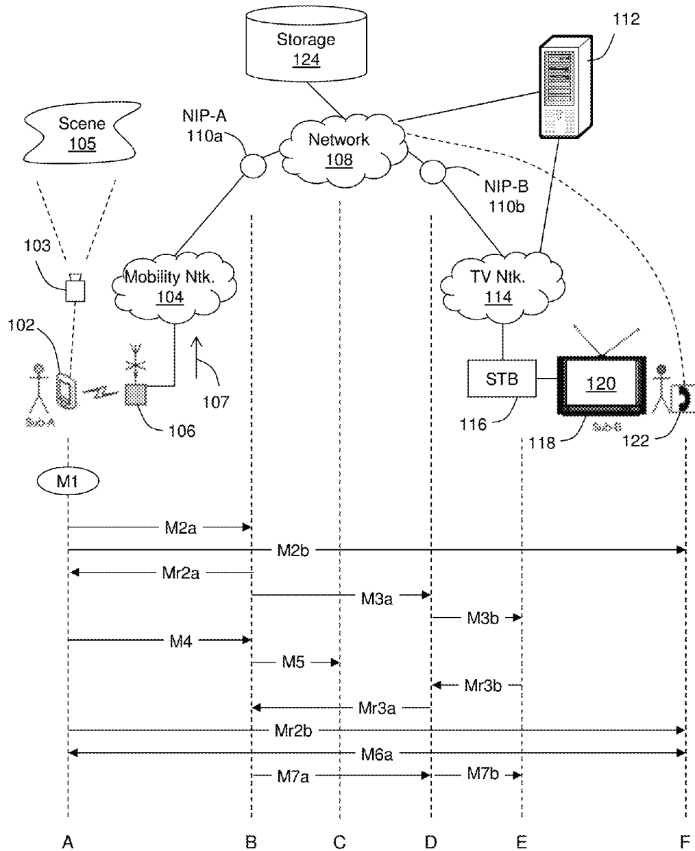
100 FIG. 1
