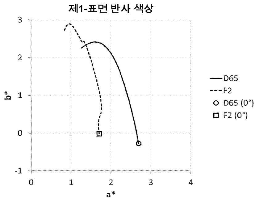
도면18
