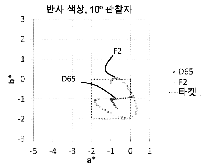
도면12
