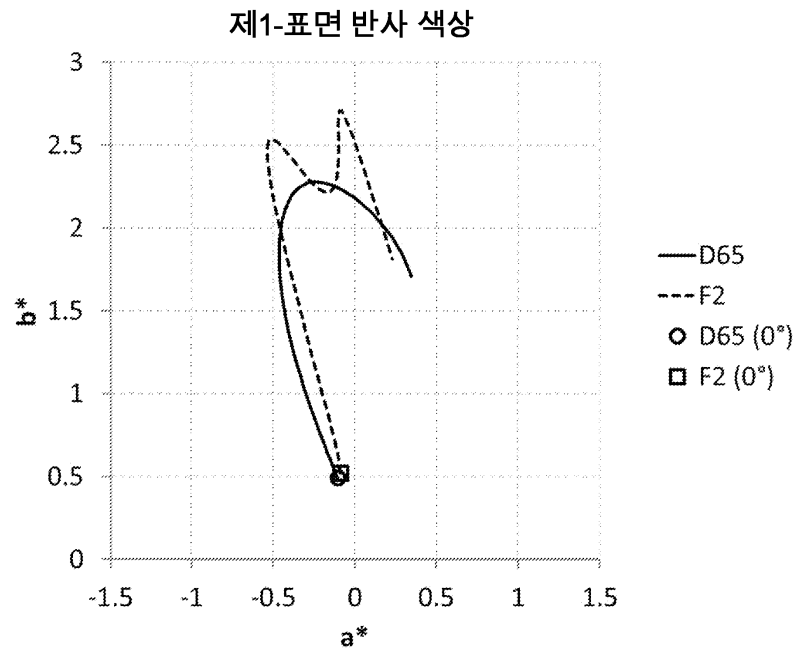
도면20
