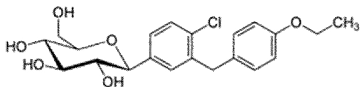
(4) Canagliflozin, dargestellt durch Formel (4):
