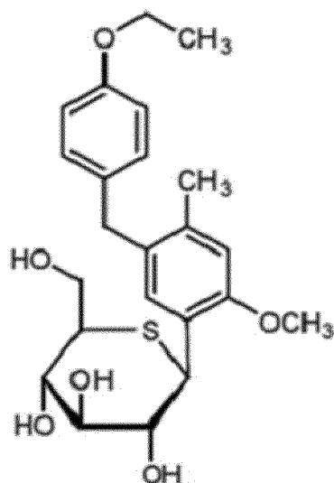
(6) Luseogliflozin, dargestellt durch Formel (6):
