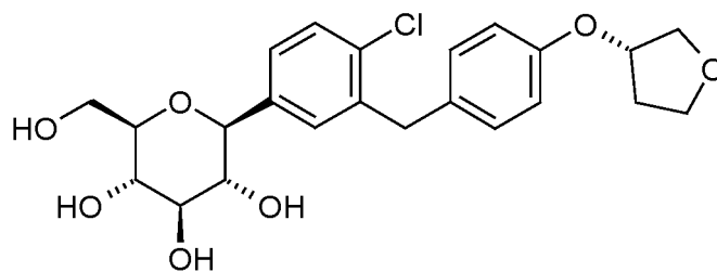
(6) Luseogliflozin, dargestellt durch Formel (6):
