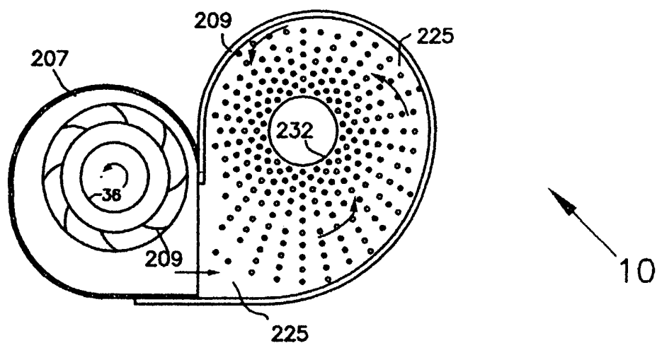
Fig. 4E View 8-8
