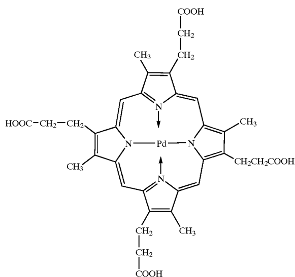
Pd COPROPORPHYRIN
