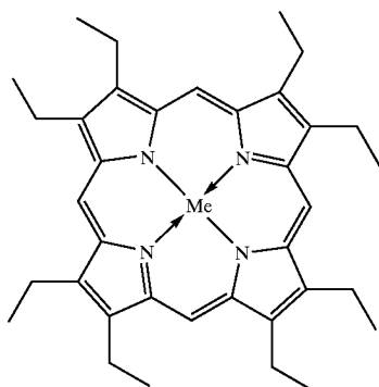
OCTAETHYLPORPHYRIN
