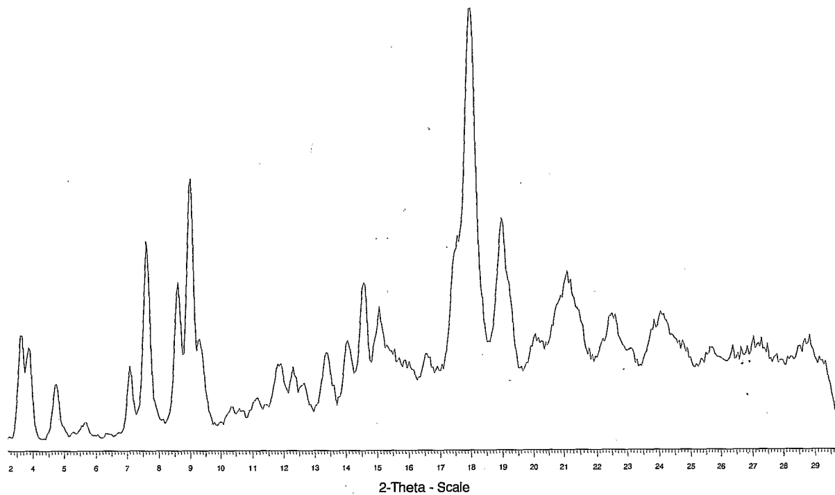
Fig. 1f XRPD of Polymorph VI (EtOAc form)
