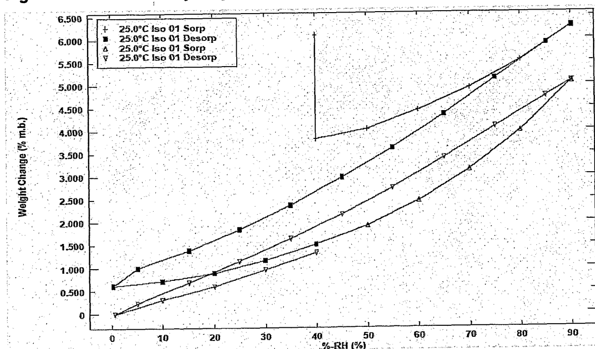
Fig. 3d GVS of Polymorph VI (EtOAc form)
