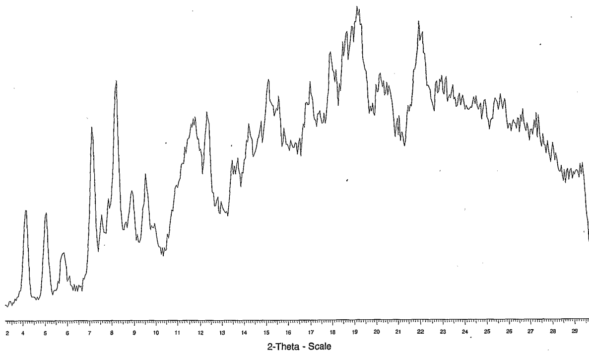
Fig. 1f XRPD of Polymorph VI (EtOAc form)
