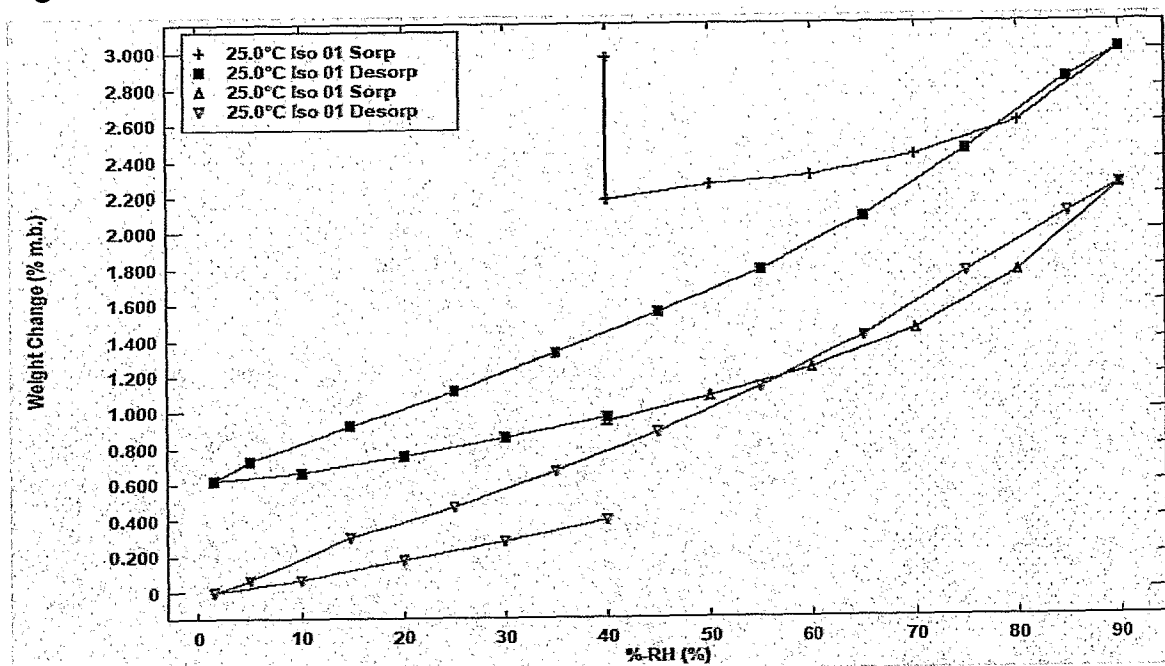
Fig. 3e GVS of Polymorph VII
