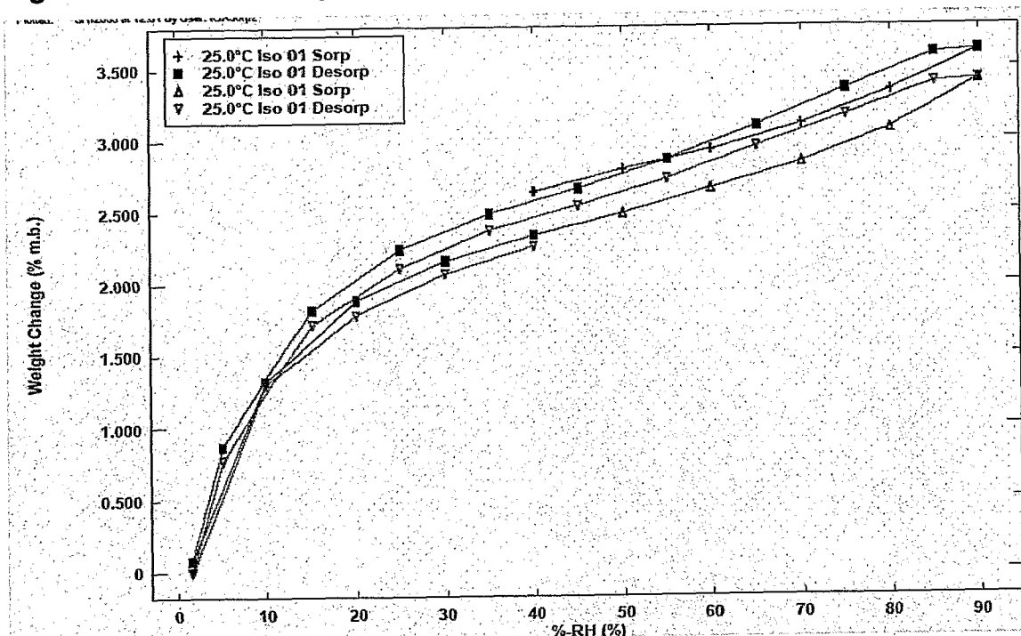
Fig. 3d GVS of Polymorph VI (EtOAc form)
