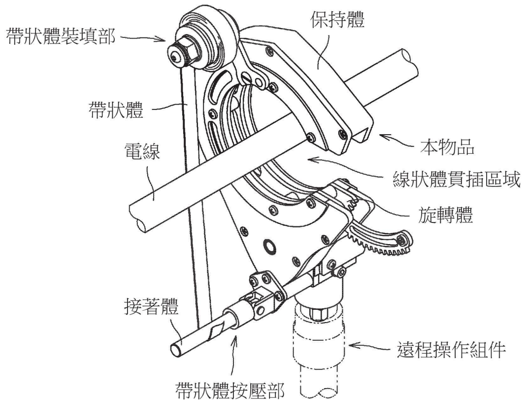
【使用狀態參考圖2】
