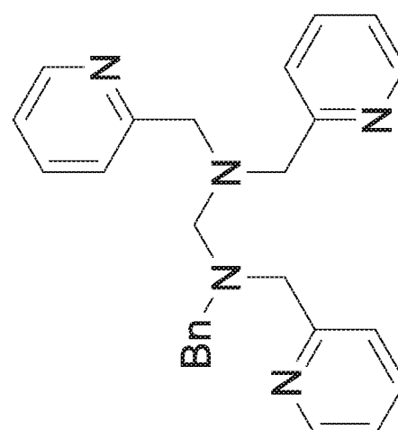
Bn-TPEN
