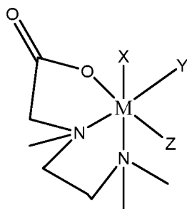
Formula VI.
