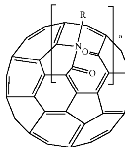
Ketolactam
