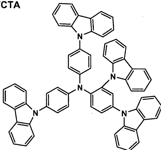
\alpha -NPD
