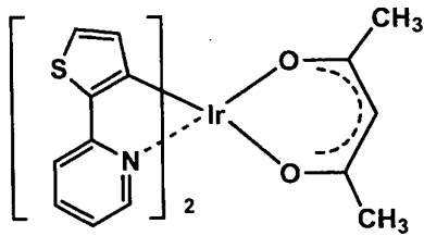
Ir-5
