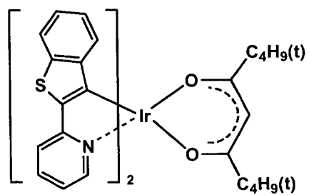
Ir-6
