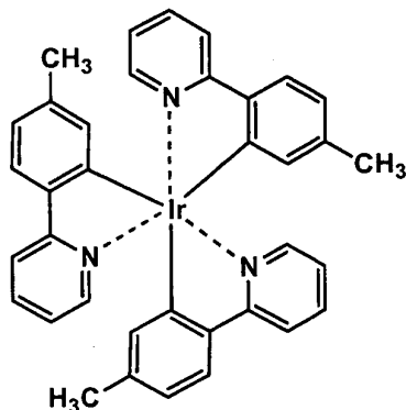
Ir-2
