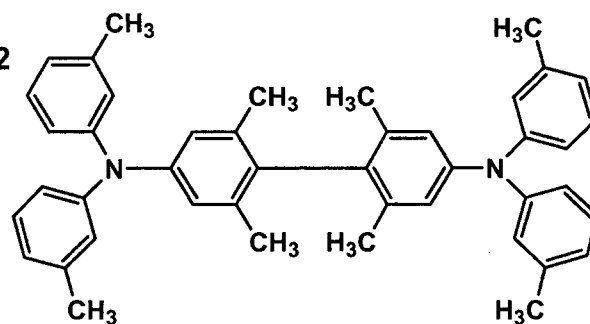
m-MTDATXA
