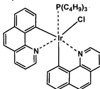
Ir-4
