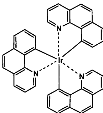
Ir-3
