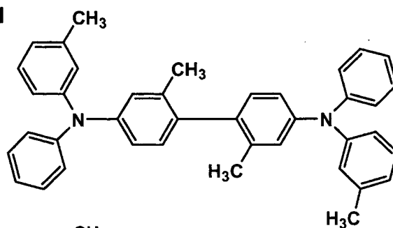
HMTPD
