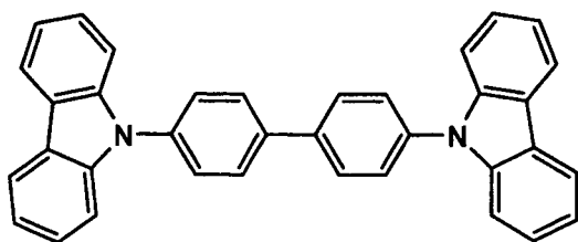
CBP
