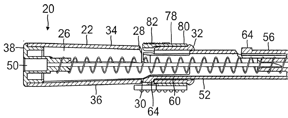
FIG. 6 SECTION D-D
