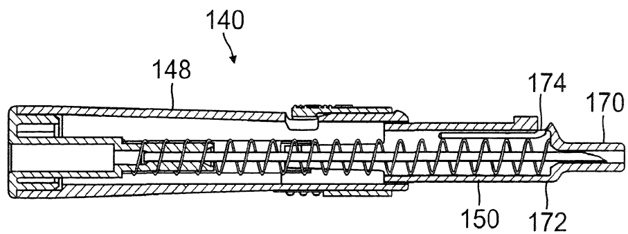
FIG. 19 SECTION D-D
