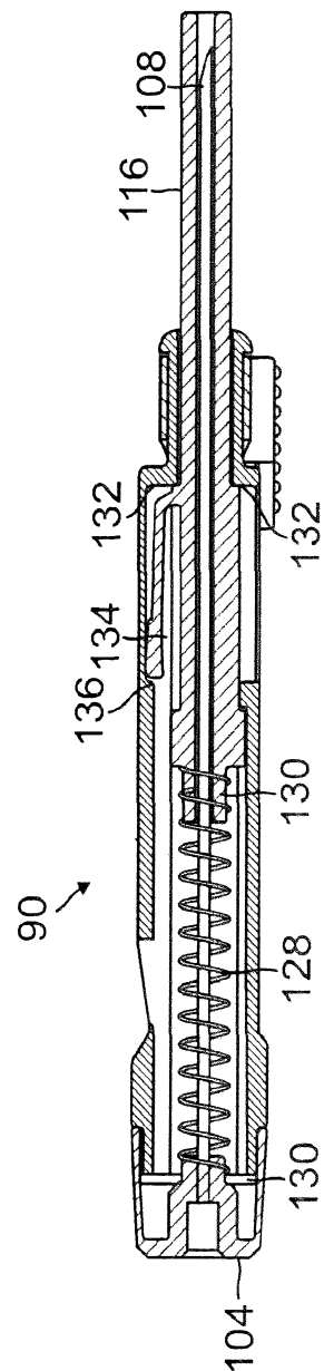
FIG. 12 SECTION D-D
