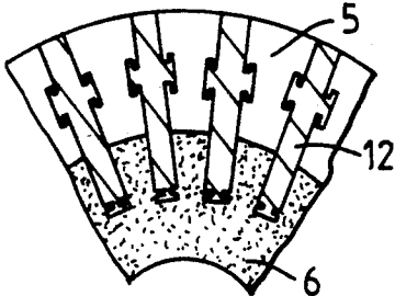
FIG. 18d
