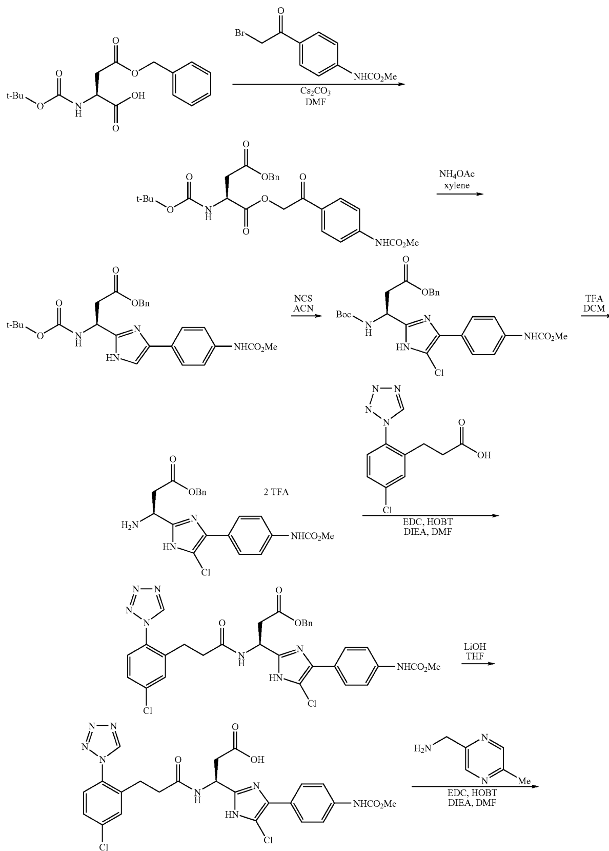
Scheme 10A
