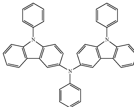
PCzPCA1
