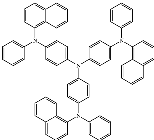
1'-TNATA
