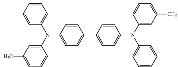
TPD
