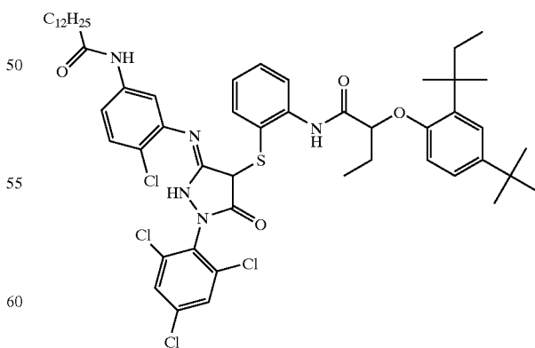
Coupler M1
