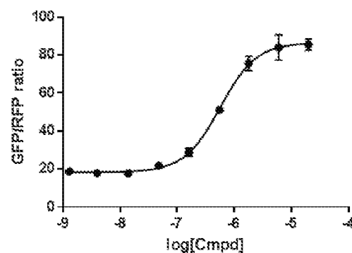
FIG. 9B Lenalidomide
