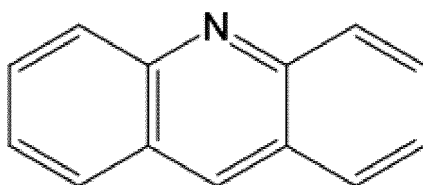
Acridine
