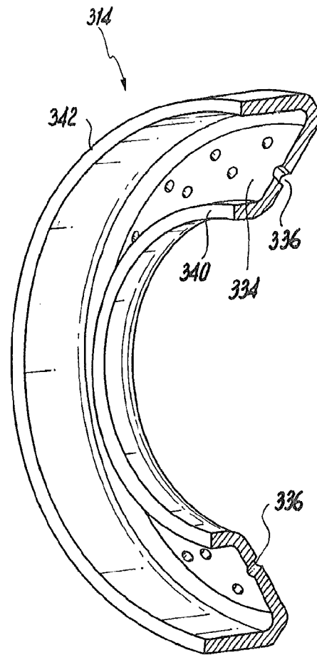
Fig. 33
