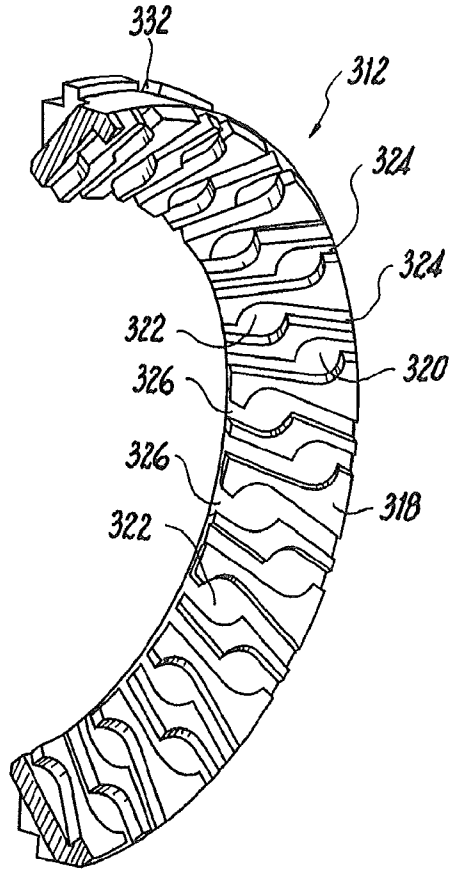
Fig. 30
