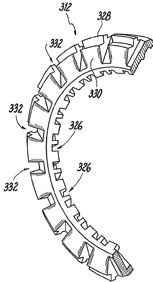
Fig. 31
