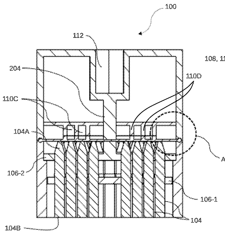
FIG. 1C
