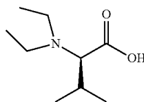
Cap-72
