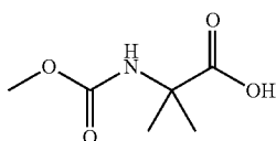
Cap-61
