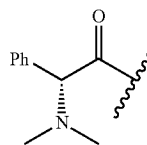
Cap-1
