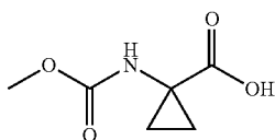
Cap-60
