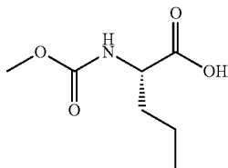
Cap-57
