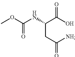
Cap-58
