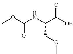
Cap-56
