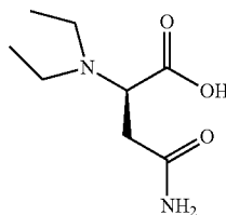
Cap-74
