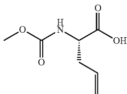
Cap-55
