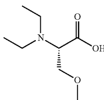
Cap-73
