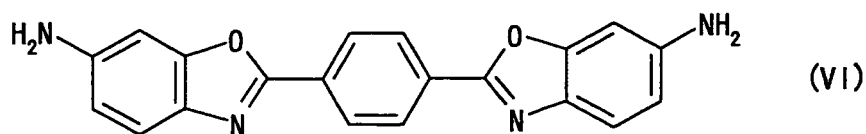
2,2'-p-phenylenebis(6-aminobenzoxazole)
