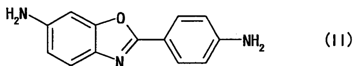
6-amino-2-(p-aminophenyl)benzoxazole
