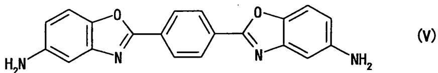
2,2'-p-phenylenebis(5-aminobenzoxazole)
