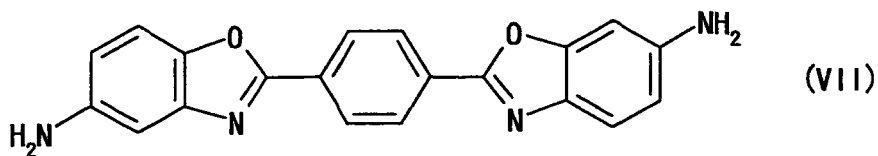
1-(5-aminobenzoxazolo)-4-(6-aminobenzoxazolo)benzene
