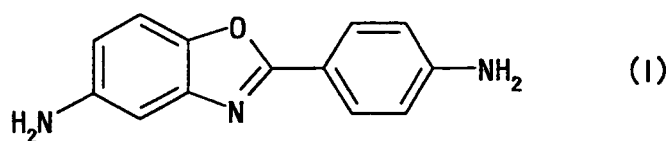
5-amino-2-(p-aminophenyl)benzoxazole
