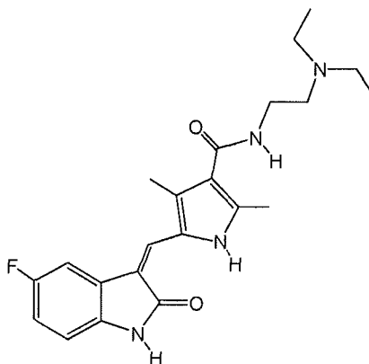
Sunitinib
