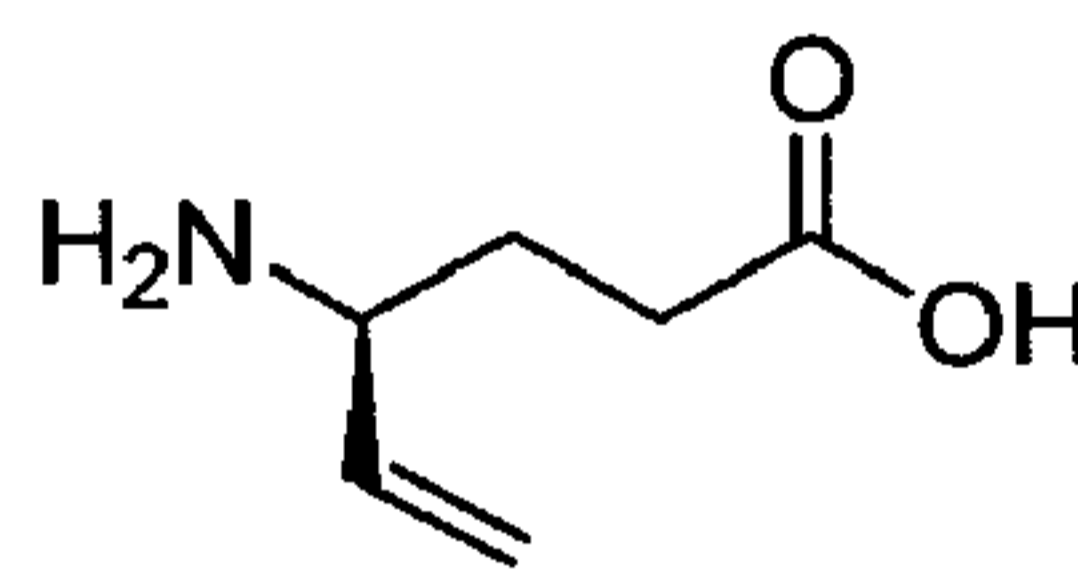
Vigabatrin-(b)
