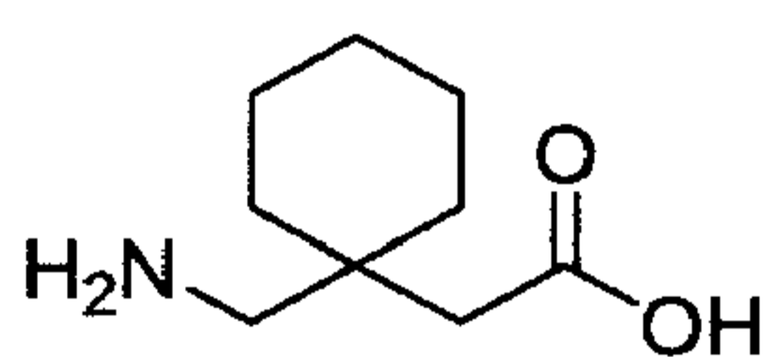
Gabapentin-(c)
