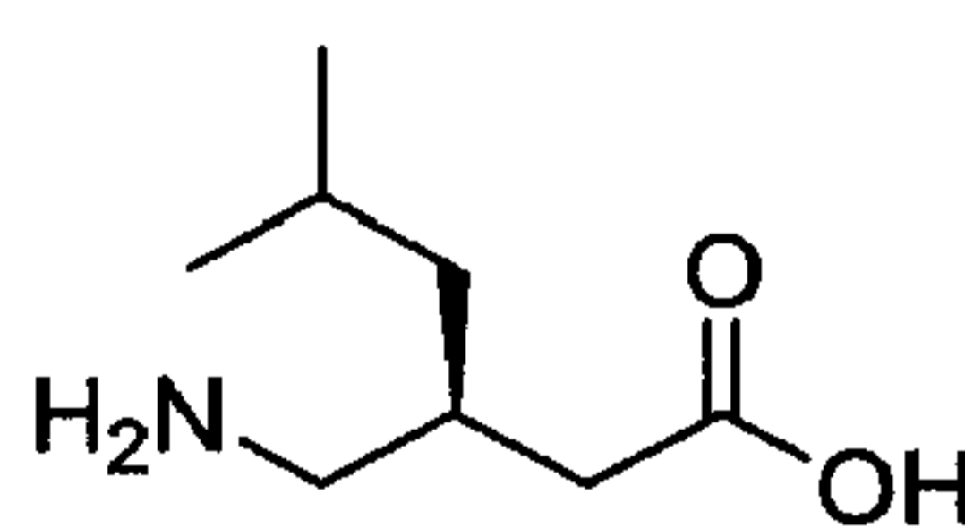
Pregabalin-(d)
