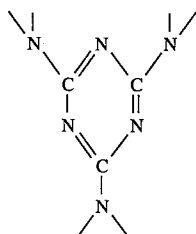
Melamine
