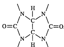
Glycoluril
