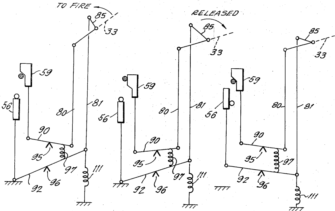
FIG. 15. FIRING
