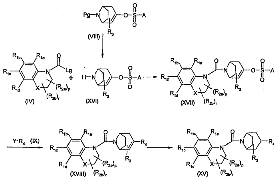
Scheme 5 (Method 2):
