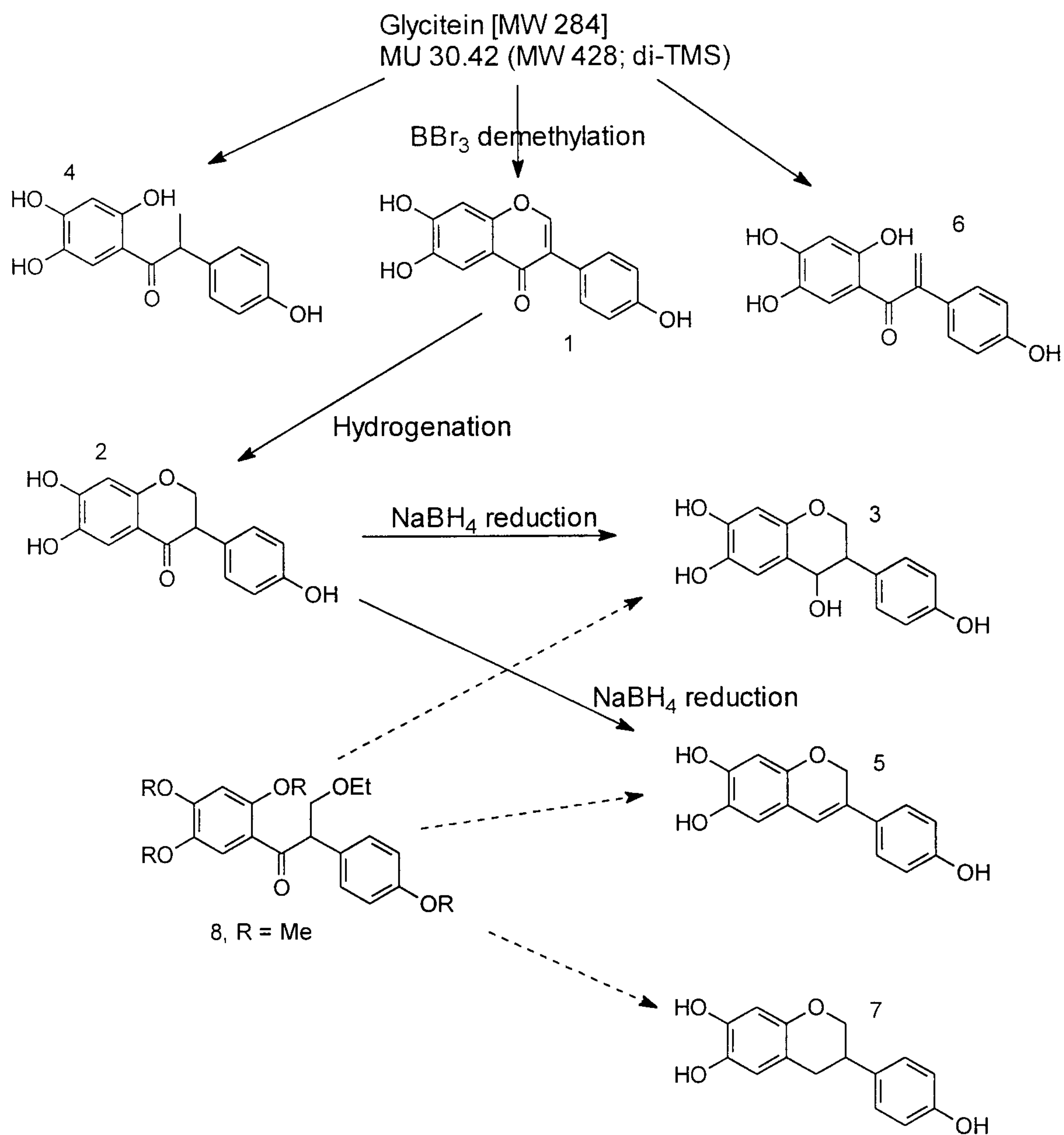
Scheme 2A
