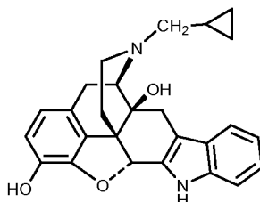
Naltrindole
