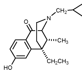
Ethylketocyclazocine (EKC)
