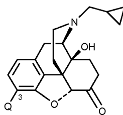
Naltrexone core
