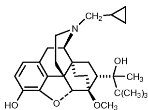
Buprenorphine
