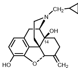
Nalmefene
