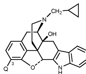
Naltrindole core
