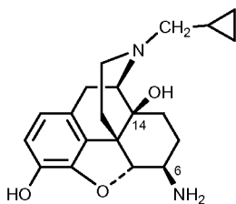
β-Naltrexamine
