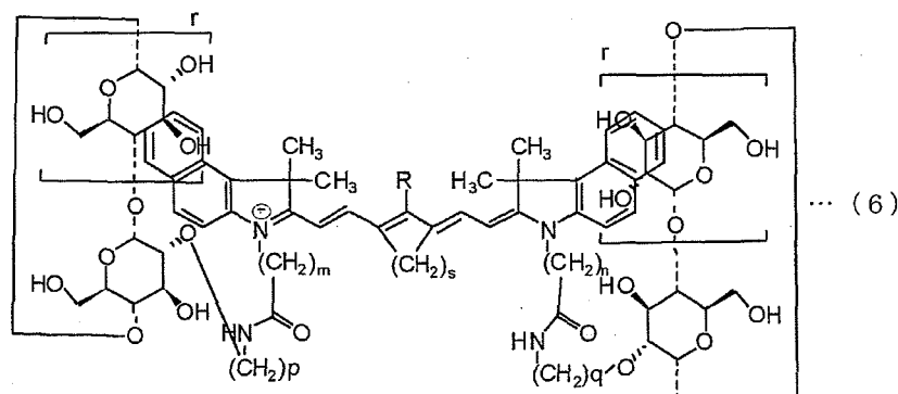
[Chem. 6]
