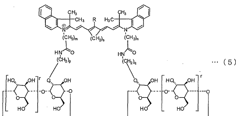
[Chem. 5]
