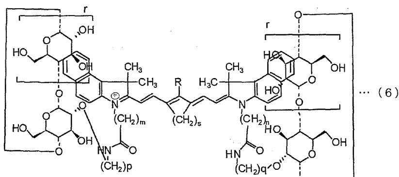
[Chem. 6]
