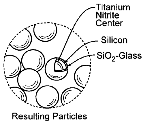
FIG. 21A
