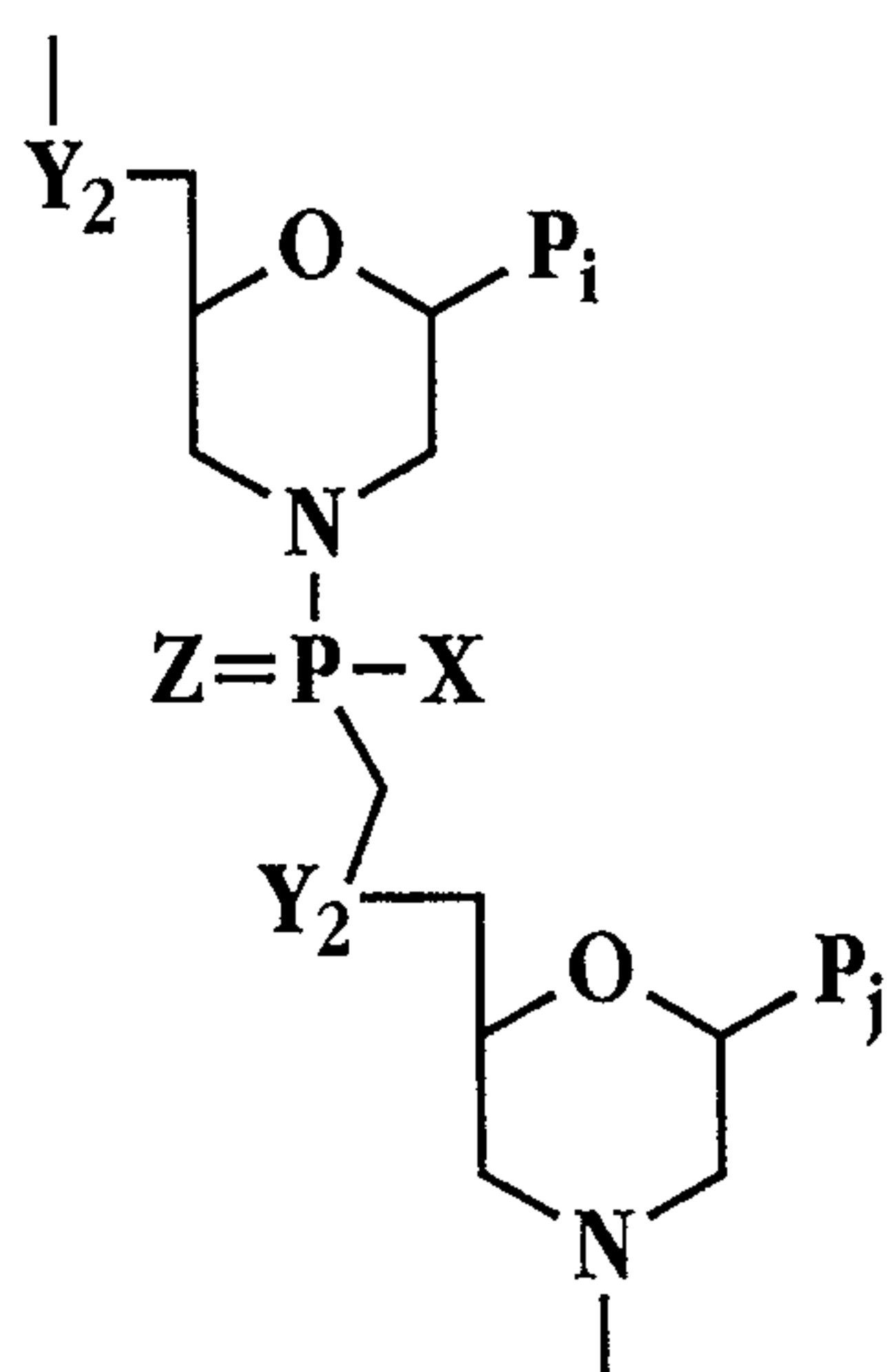
Fig. 2C-C
