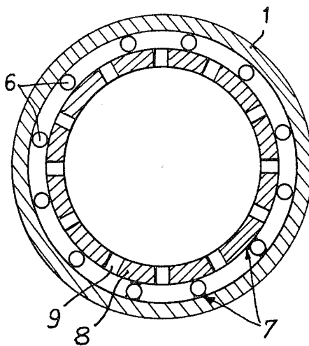
Fig:3 PRIOR ART
