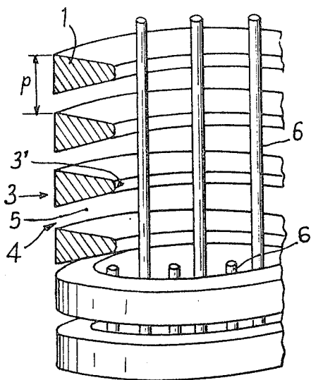
Fig:2 PRIOR ART
