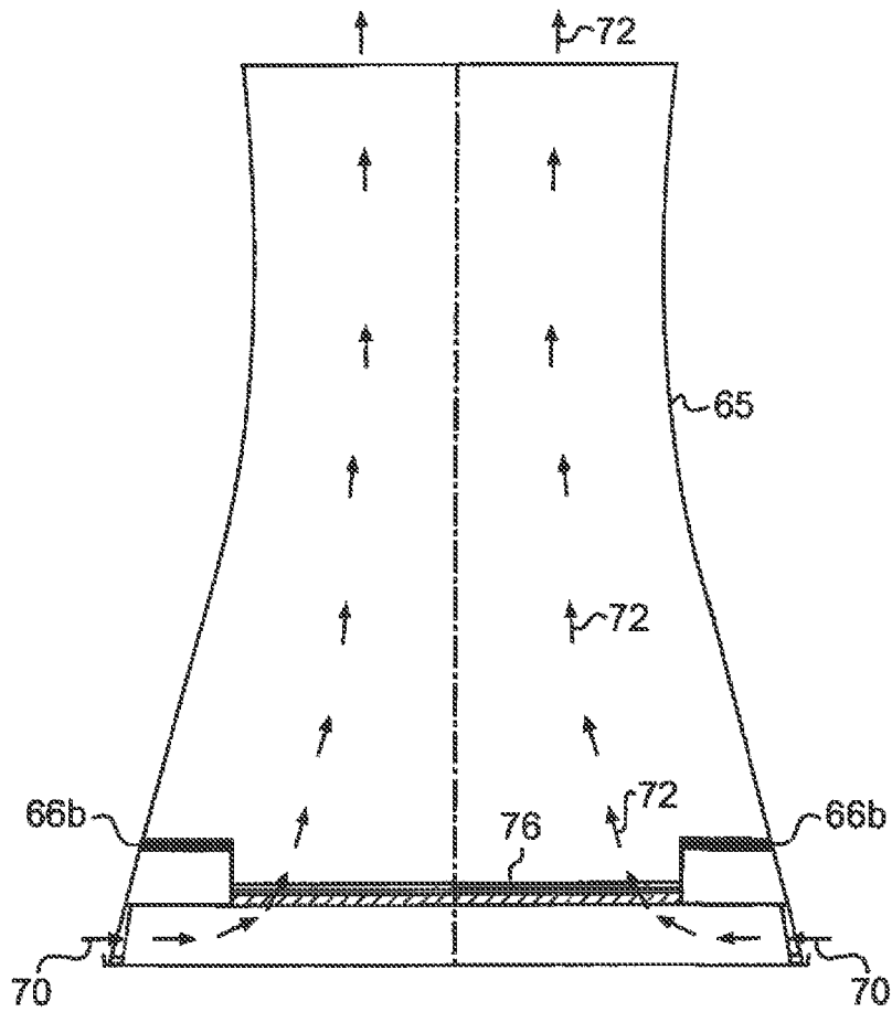
FIG. 11B
