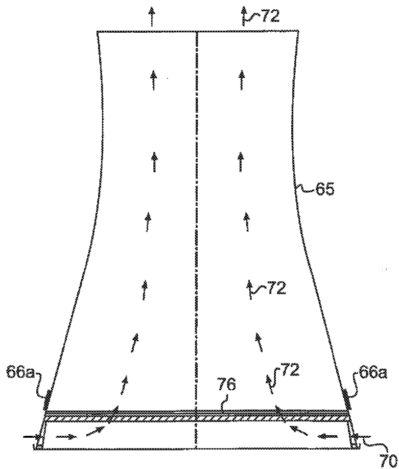
FIG. 11A
