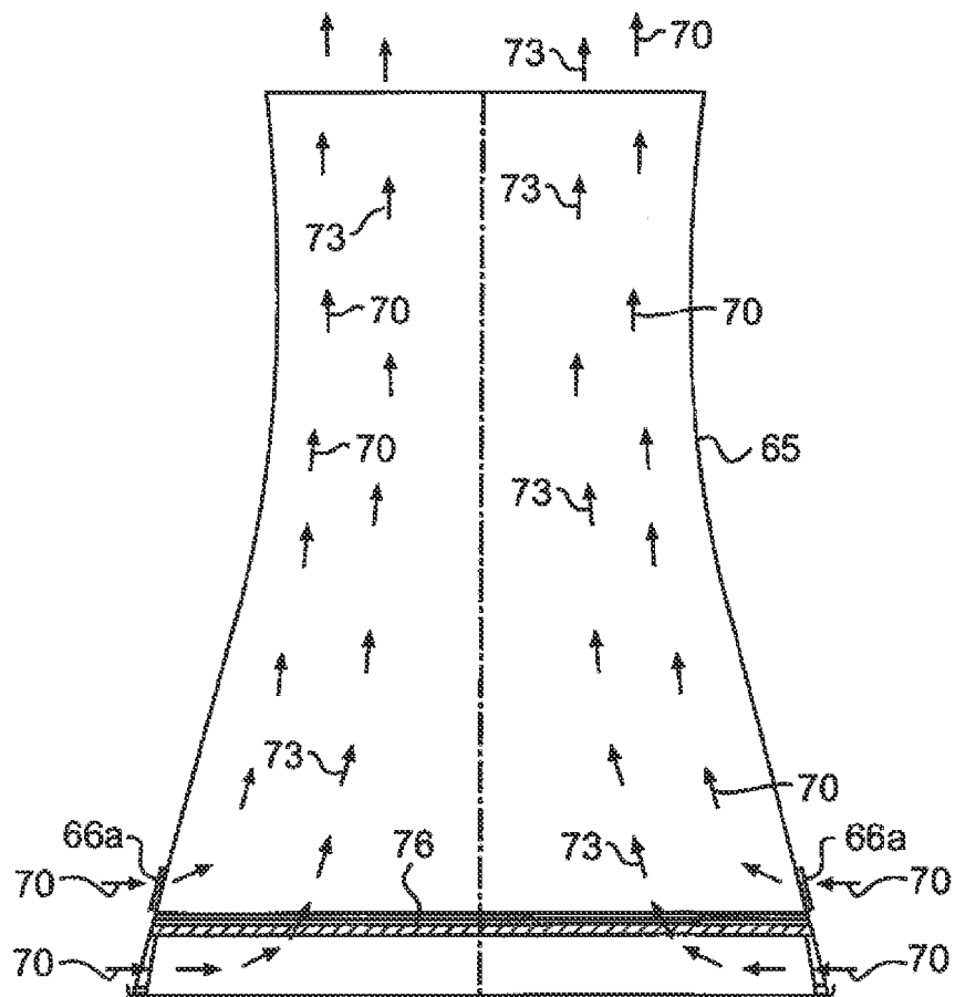
FIG. 12A
